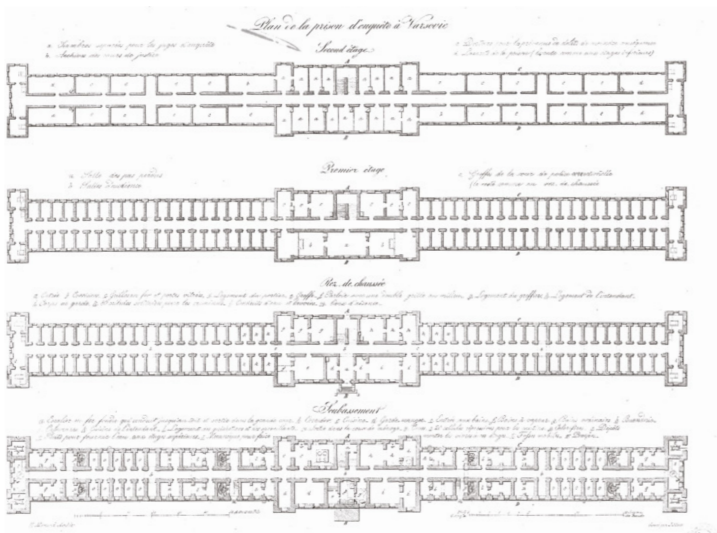
/ Rzuty parteru, pięter i poddasza więzienia śledczego w Warszawie, ze zbiorów APW /
