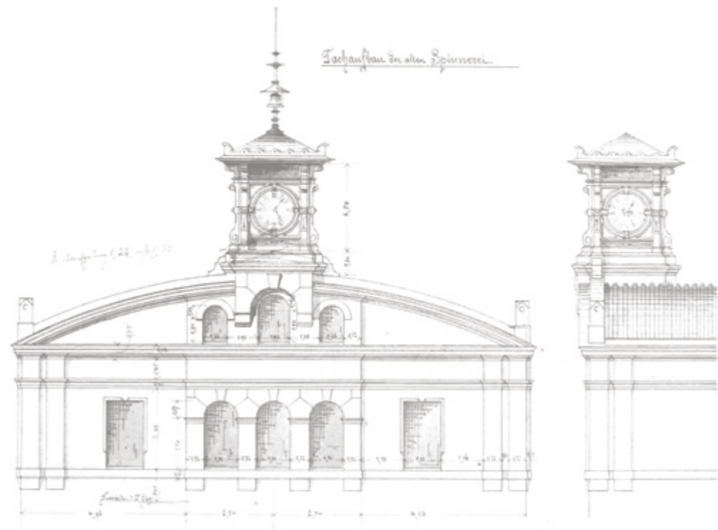
/ Wieża zegarowa i stara przędzalnia lnu w Żyrardowie – rzut i przekrój b.d., ze zbiorów APW O/Grodzisk Maz. /
