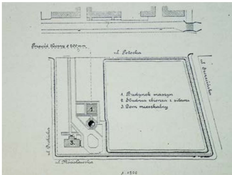
Plan Stacji Pomp Kanałowych „Żoliborz” (cyt. za: Wodociągi i kanalizacja m.st. Warszawy 1886-1936 , Warszawa 1937, s. 474-476)
